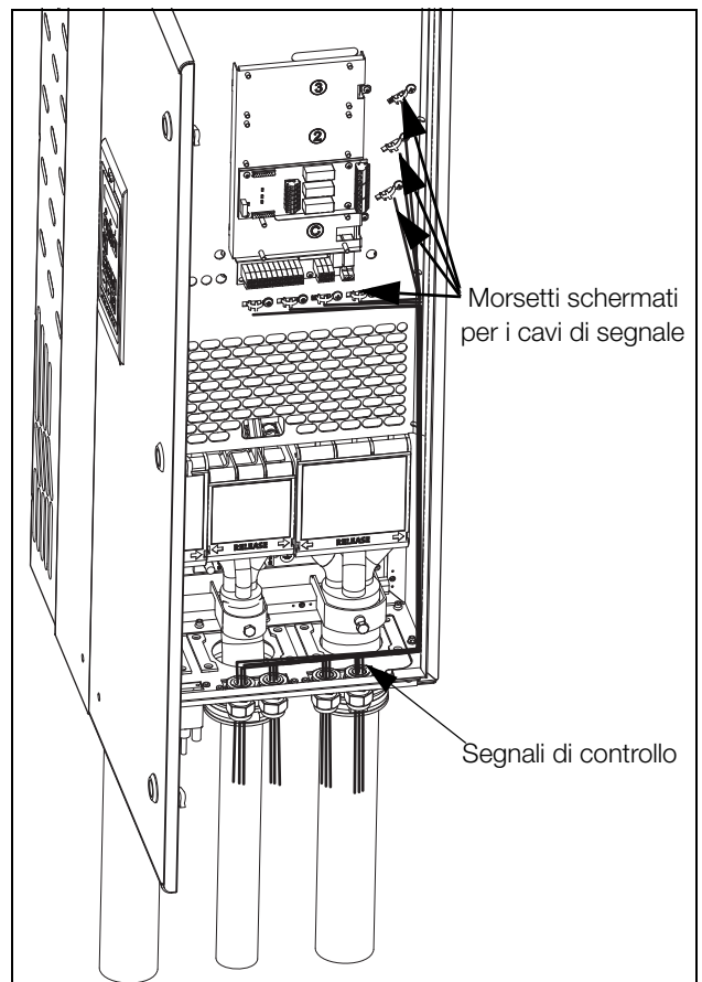
Fig. 69 Collegamento dei segnali di controllo, modelli VFX da 48-090 a 295 e modelli VFX da 69-82 a 200, formato E, F e F69 (disegno schematico).
