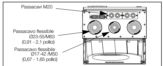
Fig. 27 Interfaccia cavi per rete elettrica, motore, CC+/CC-, resistenza di frenatura e comunicazioni, Emotron VFX modelli da 48-210 a 295 (taglia telaio F), Emotron VFX modelli da 69-082 a 200 (taglia telaio F69).
