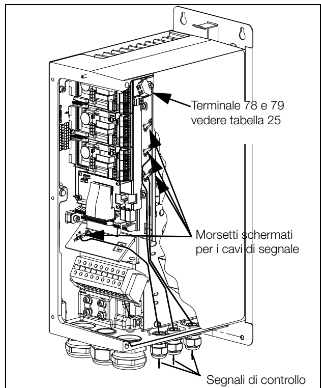
Fig. 65 Collegamento dei segnali di controllo, VFX modello da 026 a 046, formato C.
