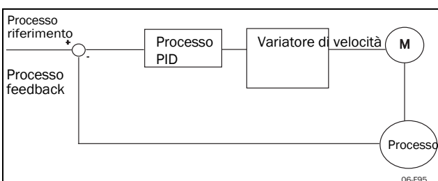
Fig. 109 Controllo PID a loop chiuso.
