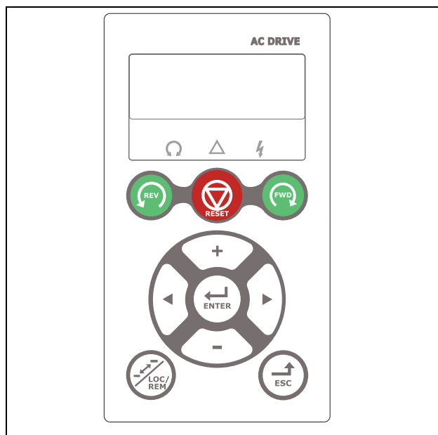
Fig. 155 Pannello di controllo con display a 4 righe.
