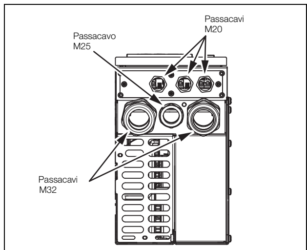
Fig. 19 Interfaccia cavi per rete elettrica, motore e comunicazioni, Emotron VFX modelli da 69-002 a 025 (taglia telaio C69).
