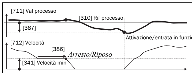
Fig. 110 Arresto/riposo PID con PID normale.
