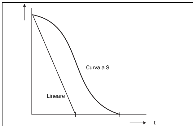
Fig. 100 Forma della rampa di decelerazione.
