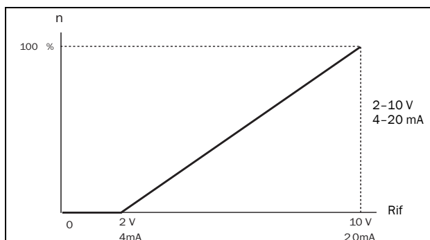
Fig. 126 2-10 V/4-20 mA (zero)
