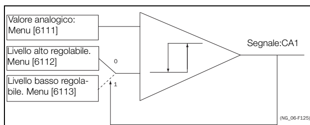
Fig. 130 Comparatore analogico con isteresi
