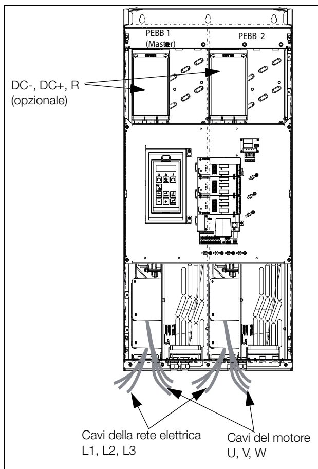
Fig. 57 Moduli IP20 formati H, H2 e G, con cavi della rete elettrica 2 x 3 e cavi del motore 2 x 3.
