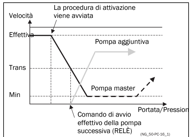
Fig. 117 Avvio con velocità di transizione
