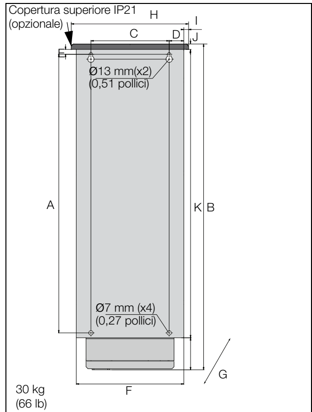
Fig. 22 Emotron VFX modelli da 48-060 a 48-105 (taglia telaio D2), modelli da 69-033 a 69-058 (taglia telaio D2(69)), vista posteriore.
