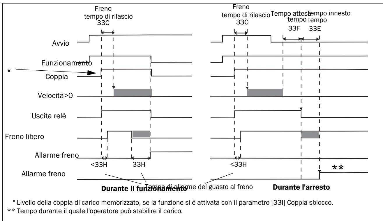
Fig. 102 Principio di funzionamento del freno per guasto durante funzionamento e arresto.
