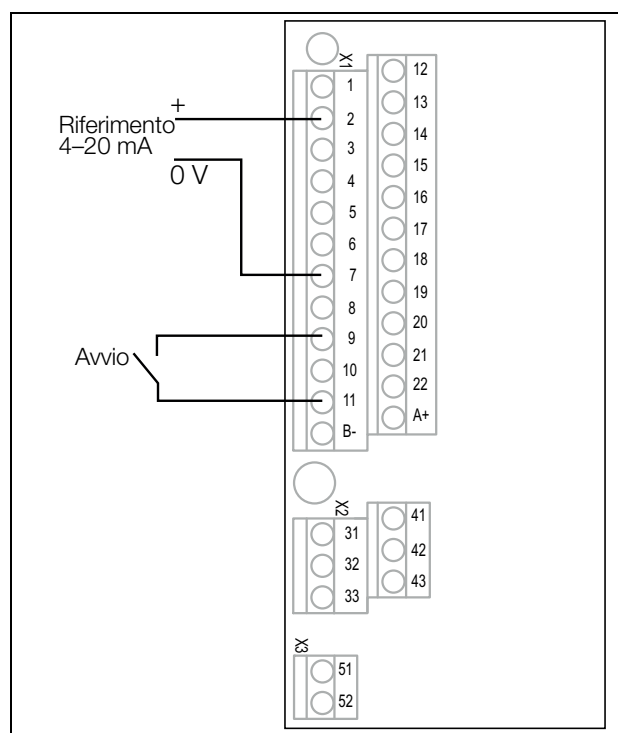
Fig. 74 Cablaggio.
