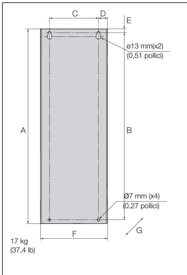
Fig. 18 Emotron VFX modelli da 69-002 a 025 (taglia telaio C69).
