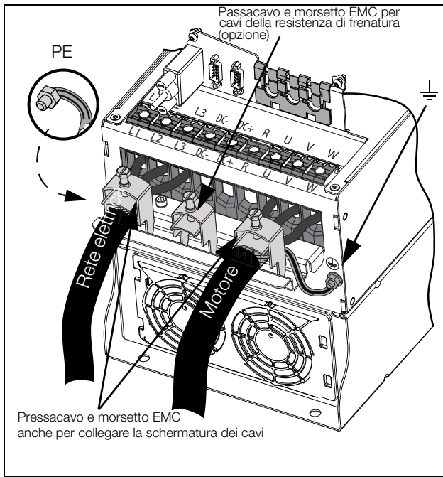
Fig. 42 Collegamenti della rete elettrica e del motore, modello da 48-060 a 48-105, formato D2 e modelli da 69-033 a 69-058, formato D2(69).
