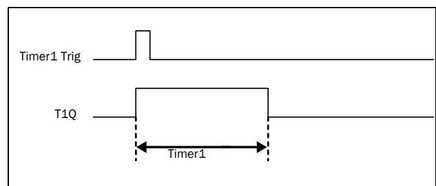
Fig. 139 Modo timer tempo di accensione.
