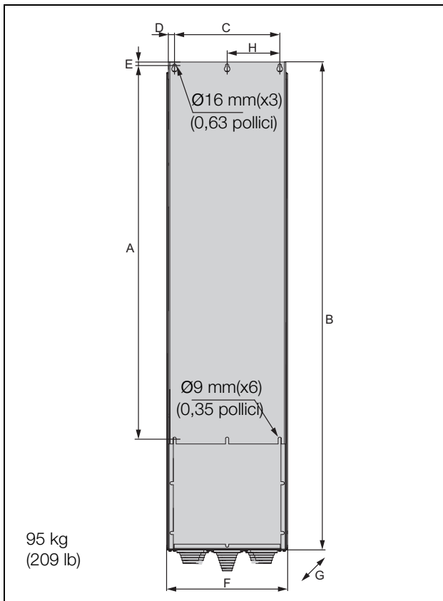
Fig. 31 Emotron VFX modello 48-365-54 (taglia telaio FA).
