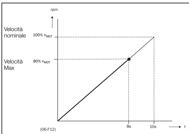
Fig. 96 Tempo di accelerazione e velocità massima.
