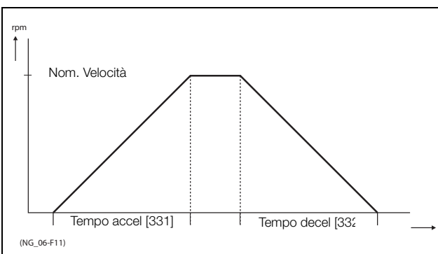
Fig. 97 Tempi di accelerazione e decelerazione.
