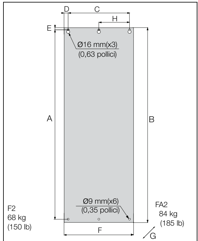
Fig. 30 Emotron VFX/ modelli da 48-205 a 48-293 (taglia telaio F2) e 48-365-20 (taglia telaio FA2).
