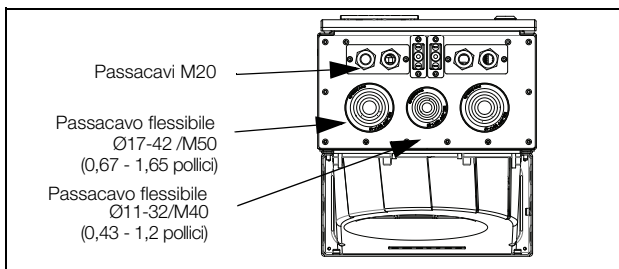
Fig. 25 Interfaccia cavi per rete elettrica, motore, CC+/CC-, resistenza di frenatura e comunicazioni, Emotron VFX modelli da 48-090 a 175 (taglia telaio E).
