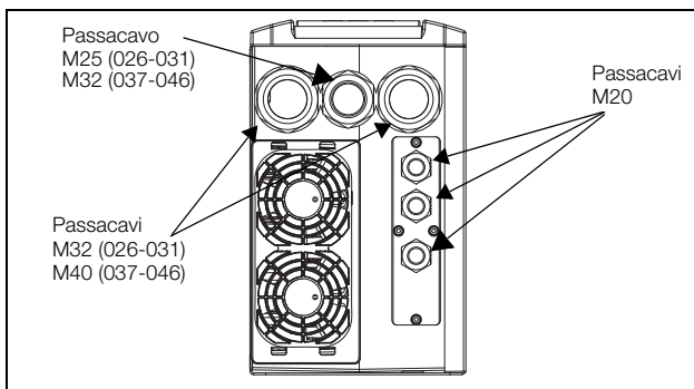
Fig. 15 Interfaccia cavi per rete elettrica, motore e comunicazioni, Emotron VFX modelli da 48/52-026 a 046 (taglia telaio C).
