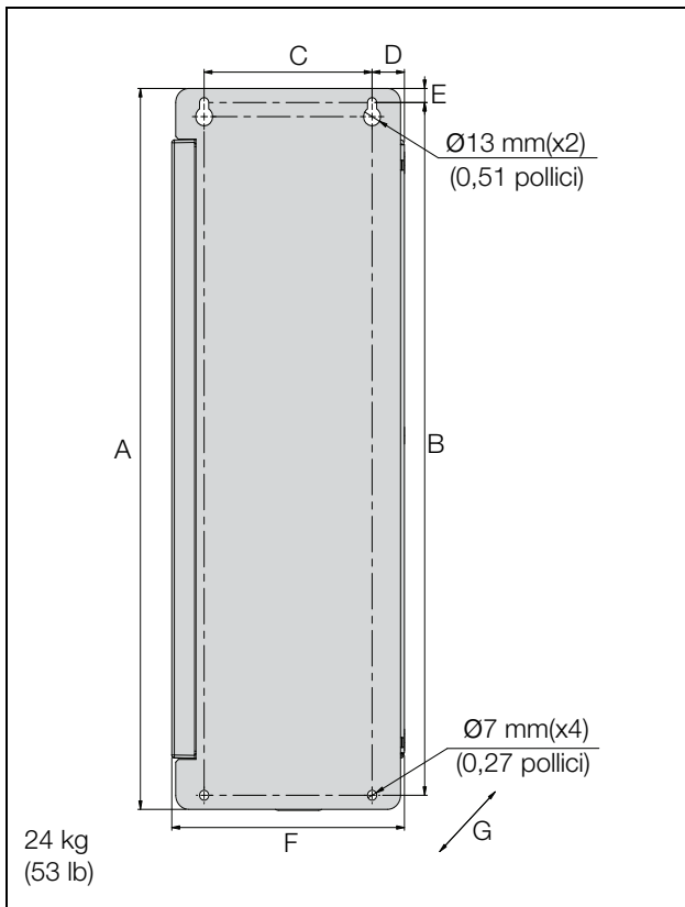
Fig. 14 Emotron VFX modelli da 48/52-026 a 046 (taglia telaio C).
