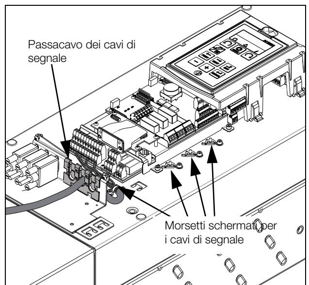
Fig. 70 Collegamento dei segnali di controllo, modelli VFX da 48-142 a 48-365, formato E2, F2 e FA2 (disegno schematico).
