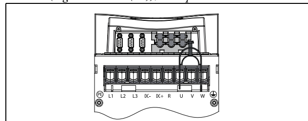
Fig. 22 Emotron VFX modelli da 48-060 a 48-105 (taglia telaio D2), modelli da 69-033 a 69-058 (taglia telaio D2(69)), vista posteriore.
