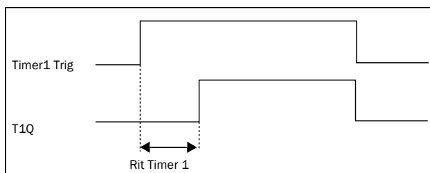
Fig. 137 Modo timer di ritardo.
