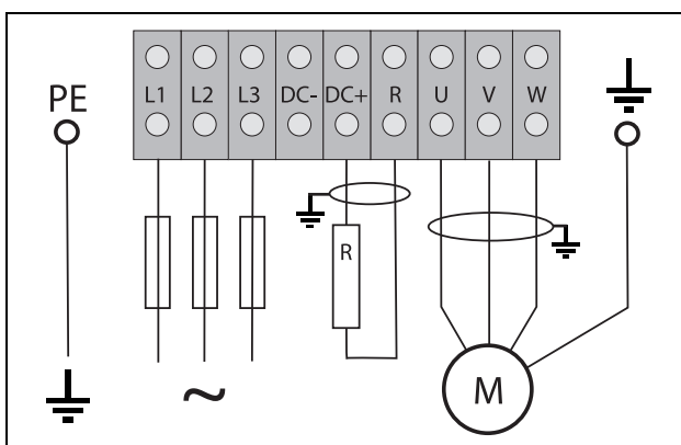
Fig. 46 L'esempio di cablaggio mostra collegamento a terra di protezione, collegamento a terra del motore e collegamento della resistenza di frenatura.
