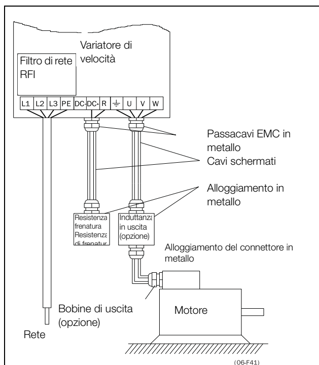
Fig. 49 Variatore di velocità stand alone.
