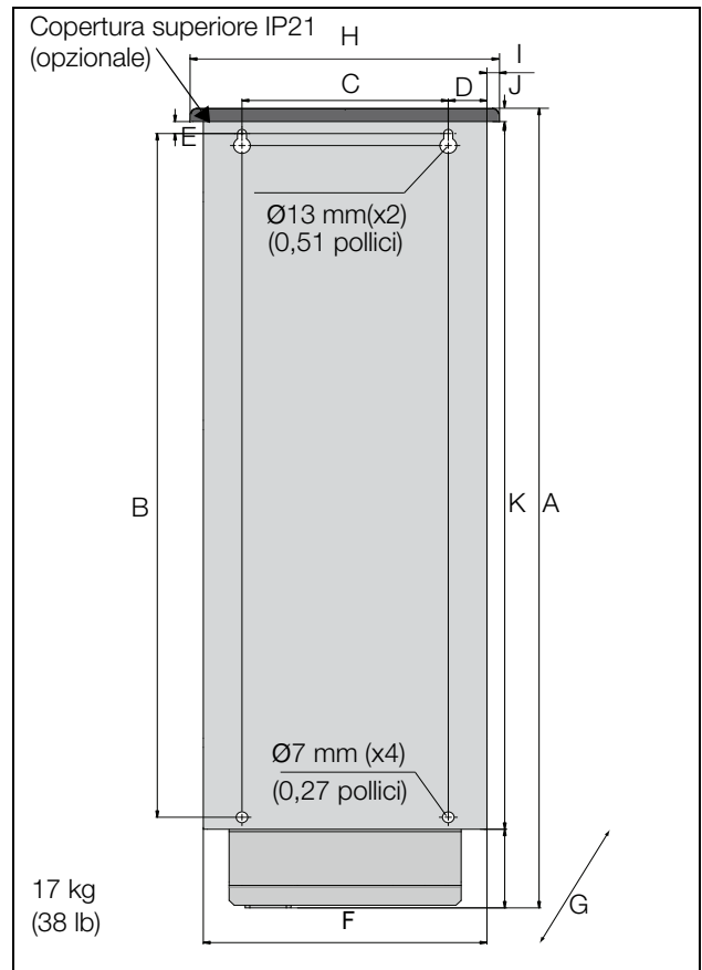
Fig. 16 Emotron VFX modelli da 48-025 a 48-058 (taglia telaio C2), modelli da 69-002 a 69-025 (taglia telaio C2(69)), vista posteriore.
