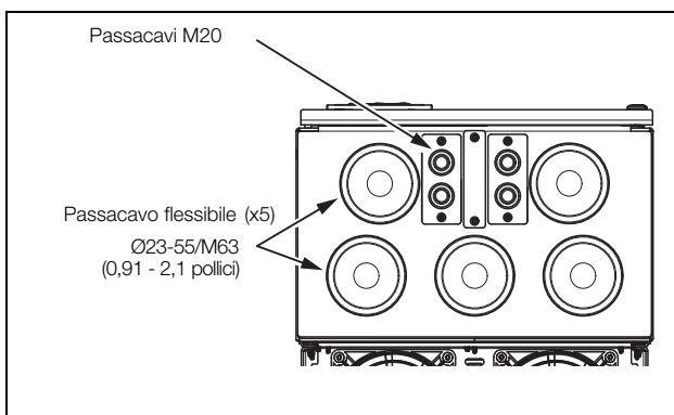
Fig. 32 Interfaccia cavi per rete elettrica, motore, CC+/CC-, resistenza di frenatura e comunicazioni, Emotron VFX modello 48-365-54 (taglia telaio FA).
