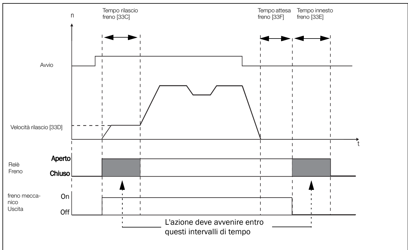
Fig. 101 Funzioni di uscita freno.
