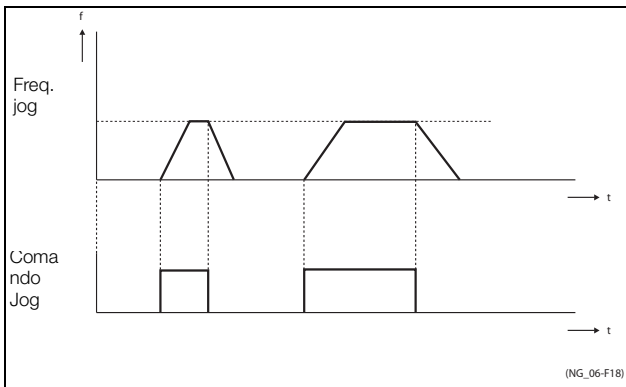
Fig. 105 Comando Jog.
