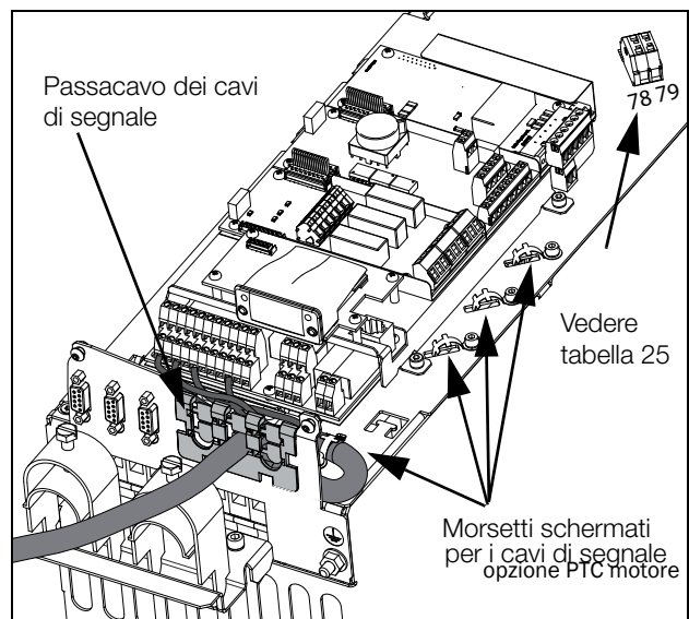
Fig. 66 Collegamento dei segnali di controllo, modelli VFX da 48-025 a 48-058, formato C2 e modelli da 69-002 a 69-025 formato C2(69).
