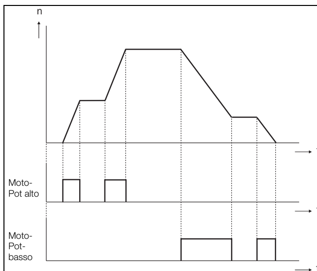
Fig. 108 Funzione Motopot.
