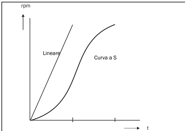
Fig. 99 Forma della rampa di accelerazione.
