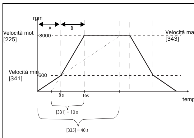
Fig. 98 Esempio di calcolo dei tempi di accelerazione (i grafici non sono proporzionali).
