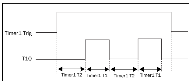
Fig. 138 Modo timer alternativo
